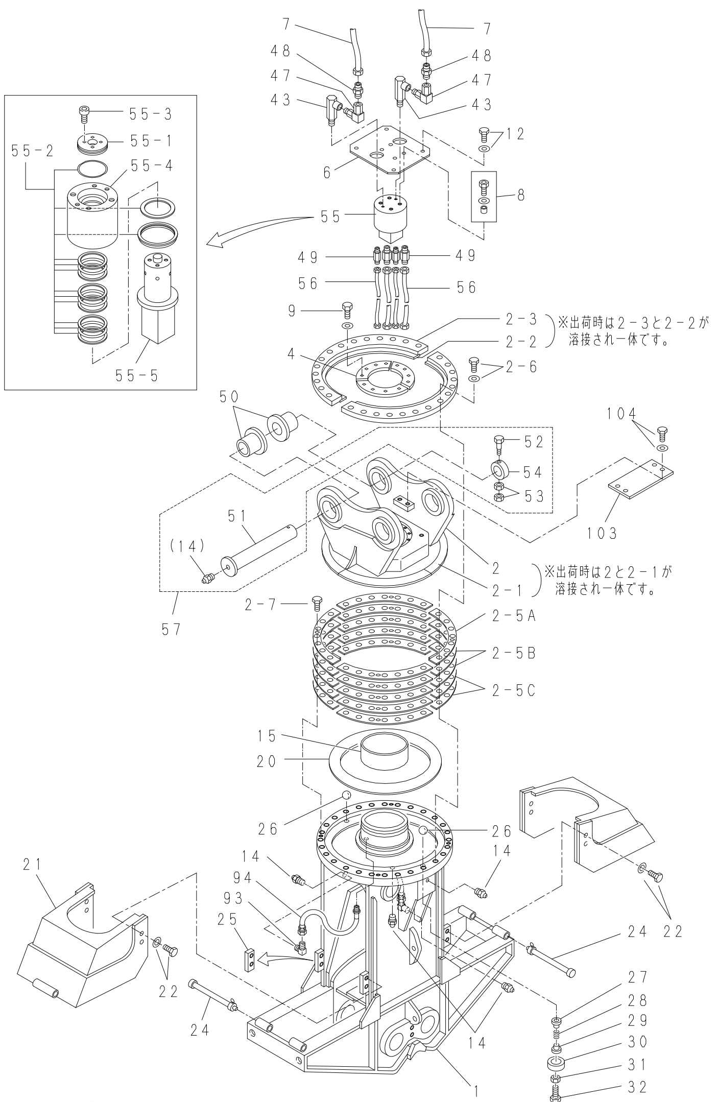
ナンデモカッター『MPCシリーズ』分解図(1/2)
